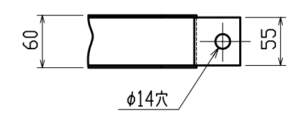
台座/脚部分詳細(S=1/6)
